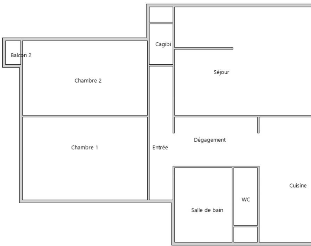
Planche (croquis) de repérage technique effectué par le cabinet : ALLODIAGNOSTIC, auteur : Boukhalafa SADALI Dossier n° 811237 du 06/10/2016 Adresse du bien : 17 RUE HENRI GUILLAUMET 478 47810A3533 77400 LAGNY SUR MARNE
